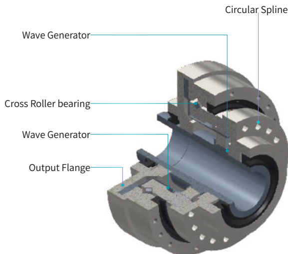
Structure of SHA Unit type /SHA유닛 타입의 구조
